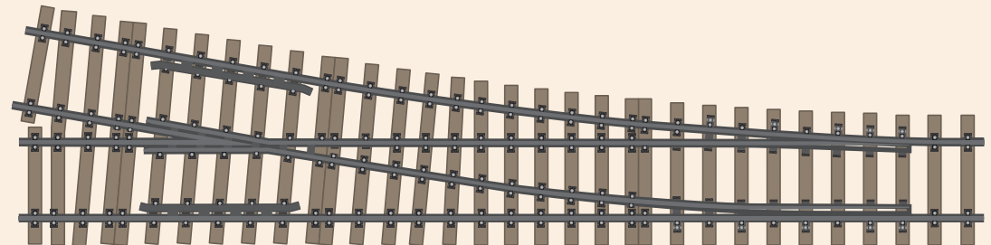
Einzelweiche rechts, 2321 mm, 10° Art.-Nr. 300305
