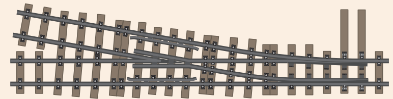
Einzelweiche rechts, ohne Antrieb, ohne Stellbock, 815 mm 10° Art.-Nr. 300381
