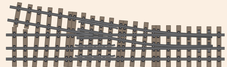
Ausweicheung rechts, ohne Antrieb, ohne Stellbock, 815 mm 10° Art.-Nr. 300385
