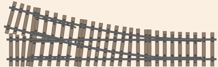
Einzelweiche rechts, 1394 mm, 15° Art.-Nr. 300301
