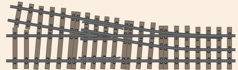
Ausfädelung rechts, ohne Antrieb, ohne Stellbock, 815 mm 10° Art.-Nr. 300383
