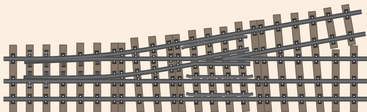
Ausweicheung links, ohne Antrieb, ohne Stellbock, 815 mm 10° Art.-Nr. 300386
